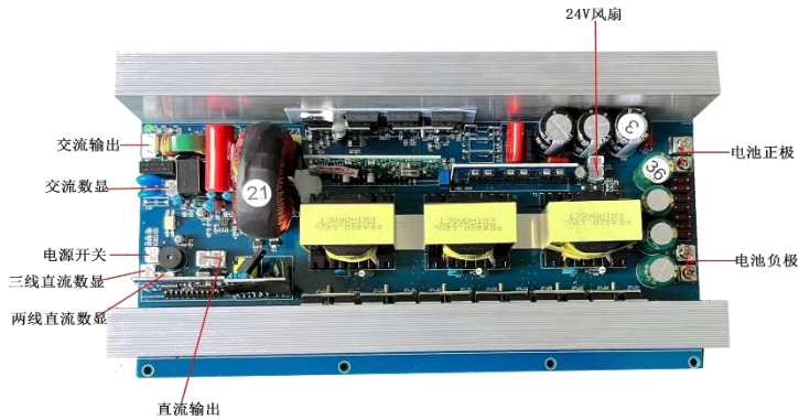
1500W接线图
